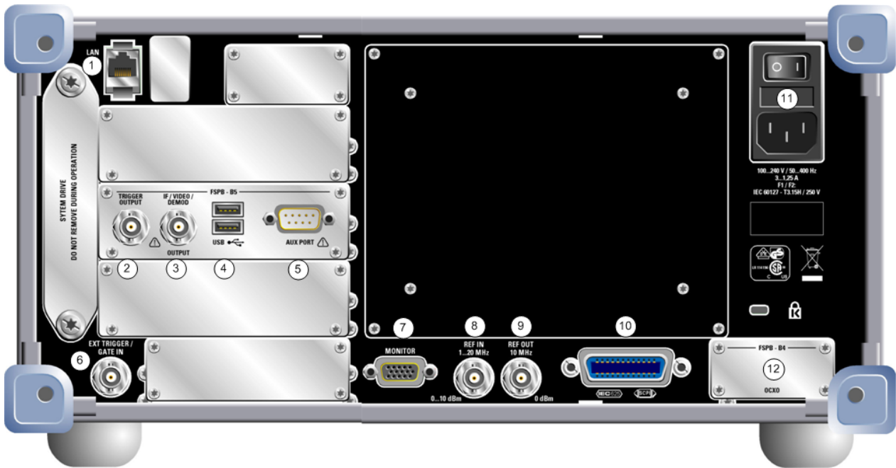
图 2-3: 后面板视图
