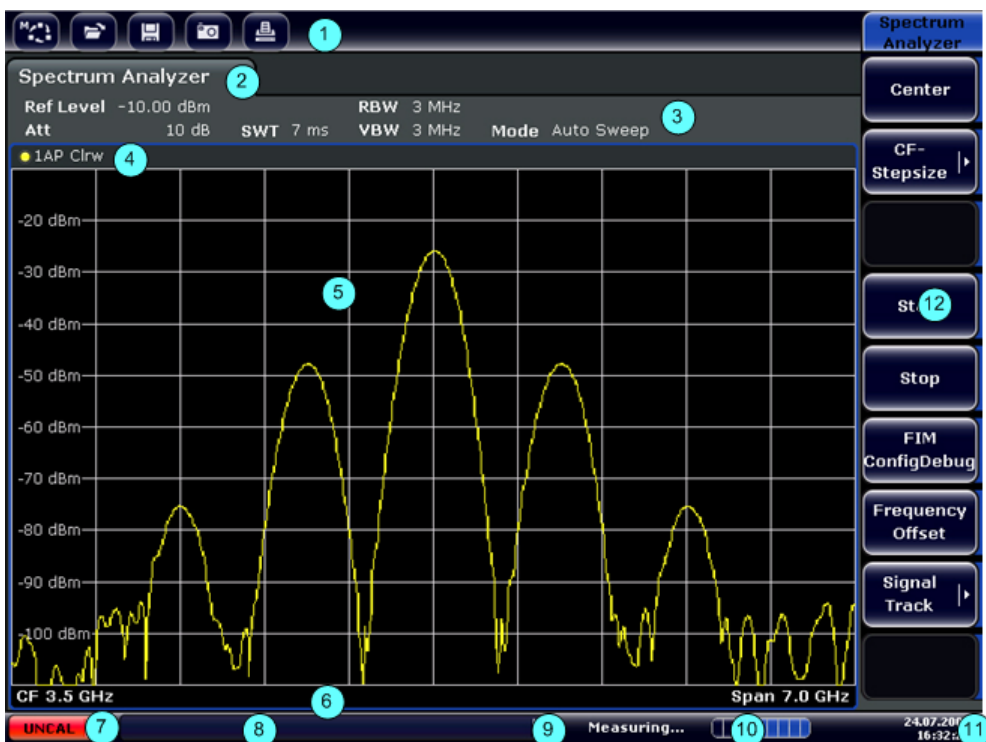
图 5-1: 分析仪操作过程中 R&SFSV 的屏幕布局
