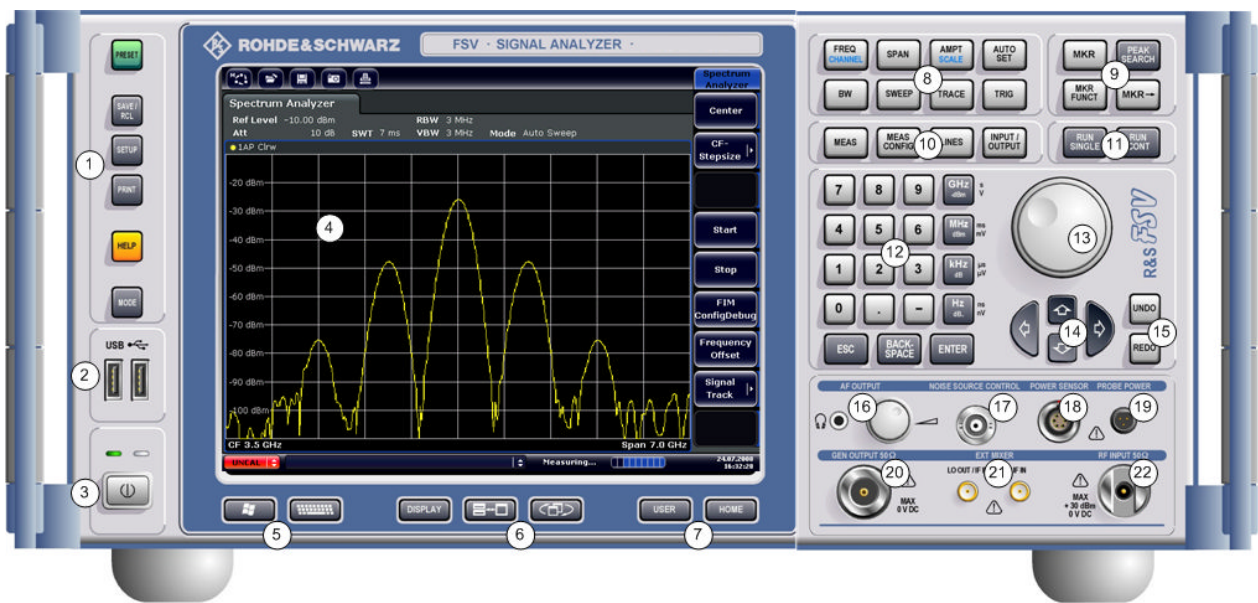
图 2-1: 前面板视图
