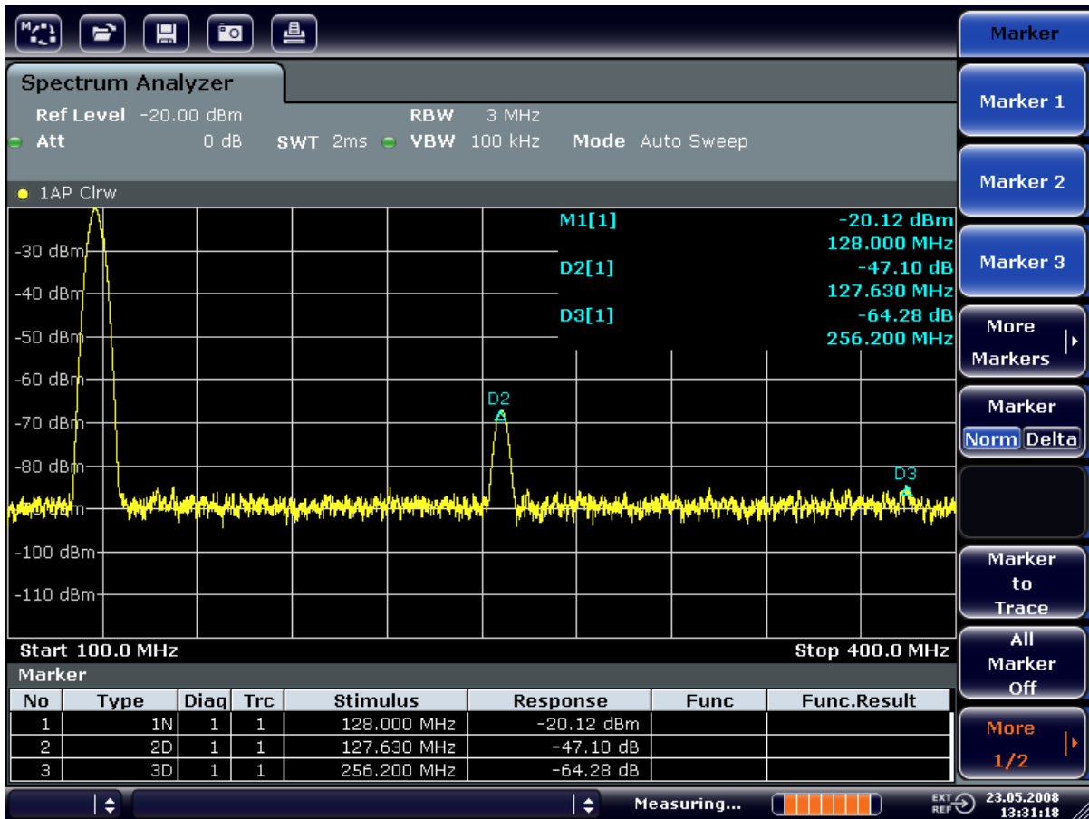
图 6-2: 测量内部参考信号发生器的谐波抑制。
